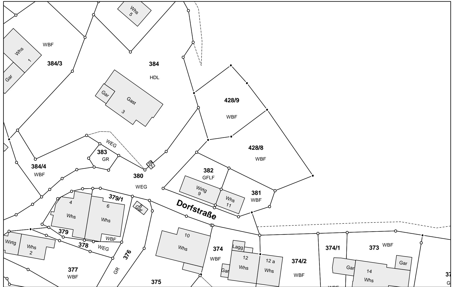
Gemeinde Bernau, Flurst.Nr. 428/9 (Kegelplatz) Lageplan Maßstab 1:750
